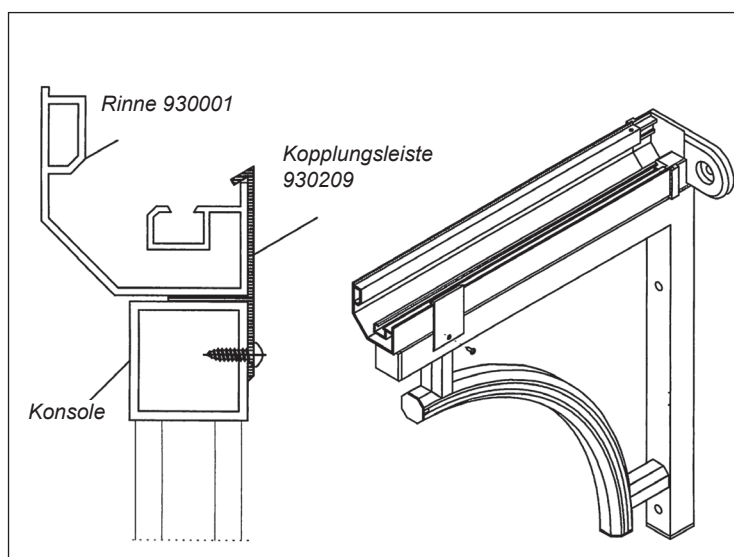
Kopplungsleiste für Vordach mit Konsole
