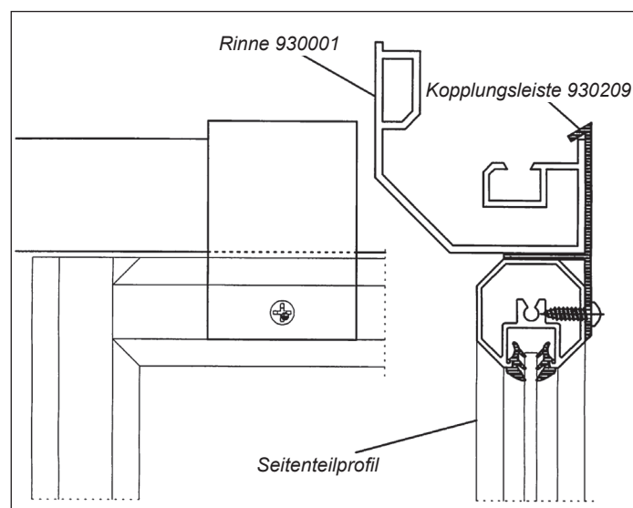
Kopplungsleiste für Vordach mit Seitenteil
